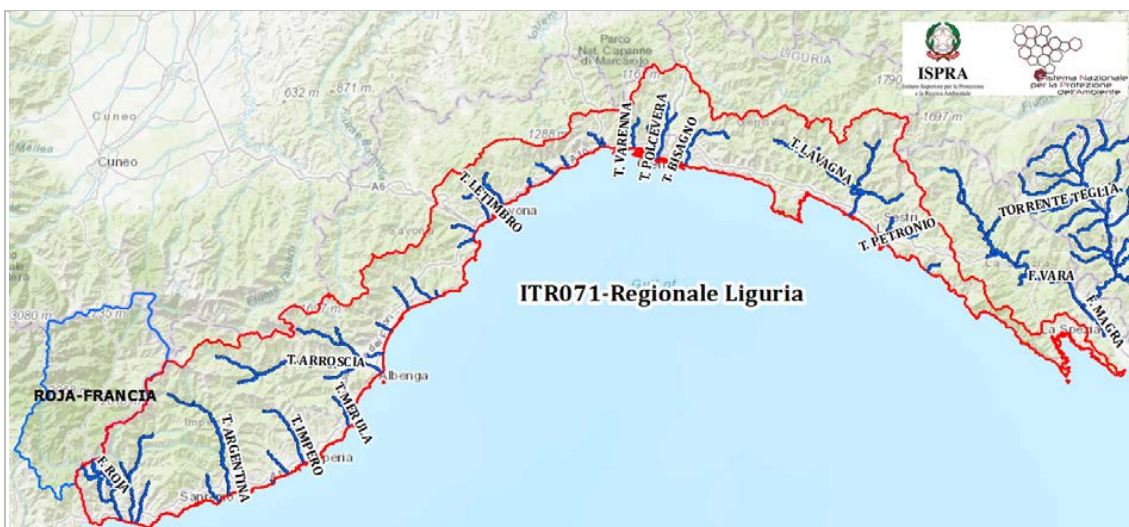
Figura 7.17 – Idrografia della UoM ITR071 (Fonte: Corpi idrici WFD – reporting WISE 2016) e porzione del bacino del Roja in territorio francese.
