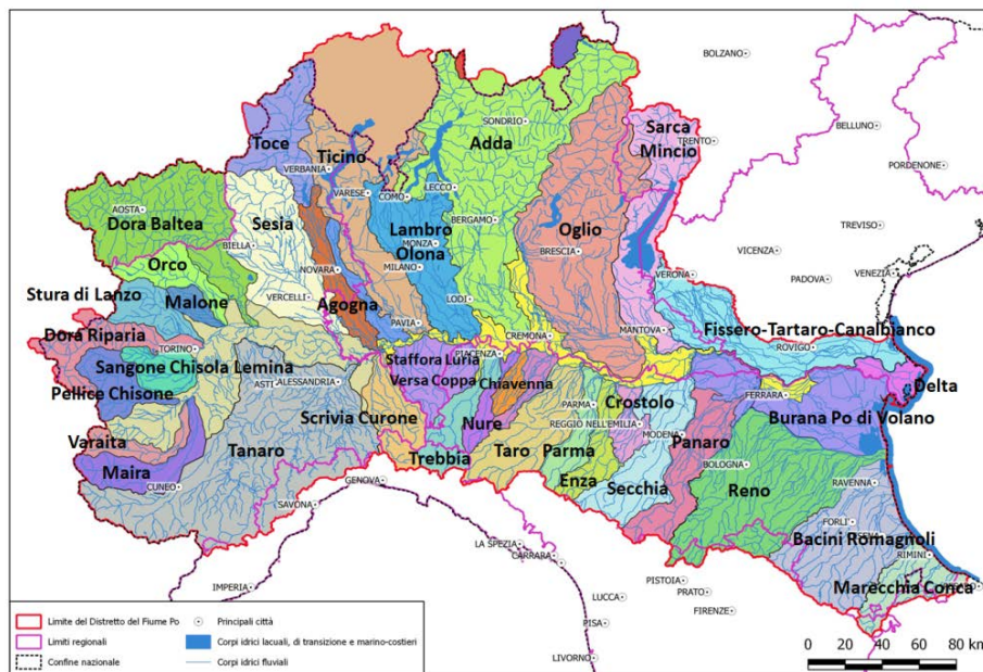
Figura 7.10 – Principali bacini e sottobacini del Distretto Idrografico del Fiume Po (Elaborazione ISPRA su immagine ABD Po).
