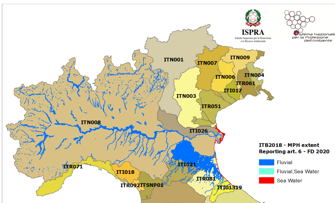
Figura 7.13 – Mappa delle aree allagabili per scenario di probabilità media ( Medium Probability Hazard – MPH) nelle UoM del Distretto Idrografico del Fiume Po differenziate per origine dell’alluvione (source = Fluvial; Sea Water; Fluvial + Sea Water) – Reporting FD 2020.
