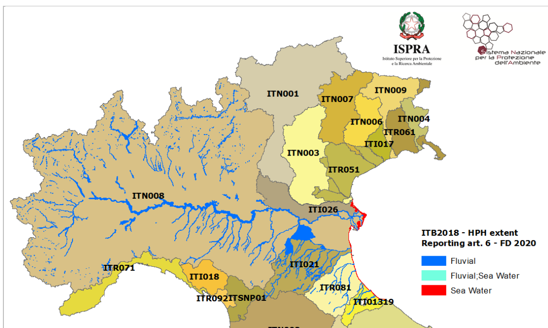
Figura 7.12 – Mappa delle aree allagabili per scenario di probabilità elevata ( High Probability Hazard – HPH) nelle UoM del Distretto Idrografico del Fiume Po differenziate per origine dell’alluvione (source = Fluvial; Sea Water; Fluvial + Sea Water) – Reporting FD 2020.
