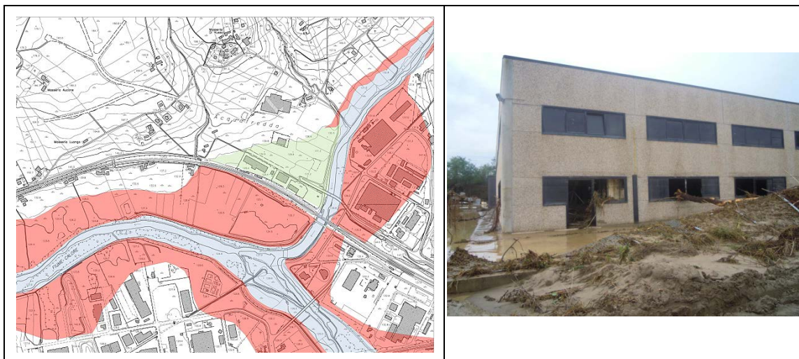
Figura 7.33 – Confluenza tra i fiumi Calore e Tammaro, in prossimità della zona industriale di Ponte Valentino (Zona ASI) nel comune di Benevento; mappa delle aree allagate (in rosso) a seguito dell’evento dell’ottobre 2015 (Fonte: ABD Appennino Meridionale, 2018) e immagine di danni provocati dall’inondazione (Fonte: Autorità di Bacino LGV, 2015).
